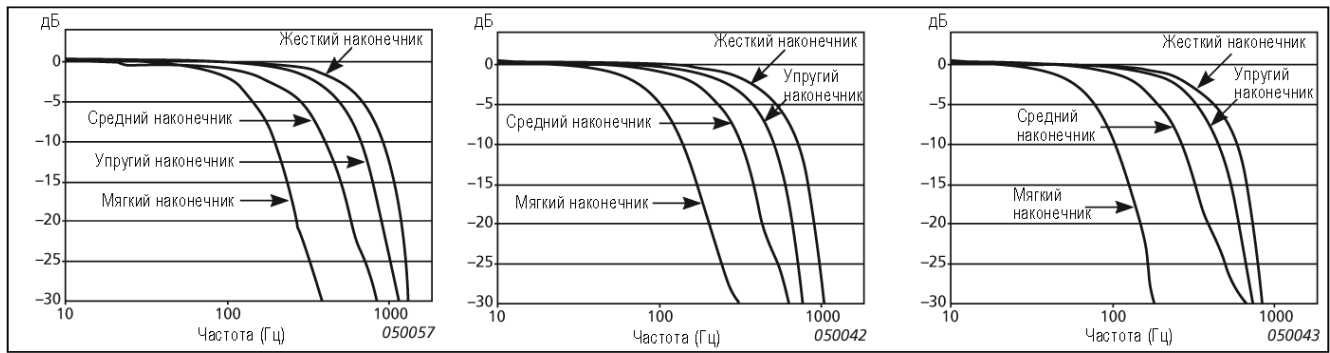
Рисунок 2. Спектр силы в виде амплитудно-частотной характеристики различных молотков и ударных наконечников. Слева направо: типы 8207, 8208 и 8210.
