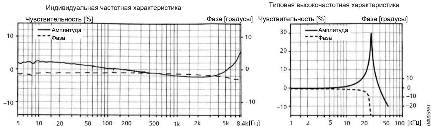
Рисунок 2. Типовая Частотная характеристика модели 4383
