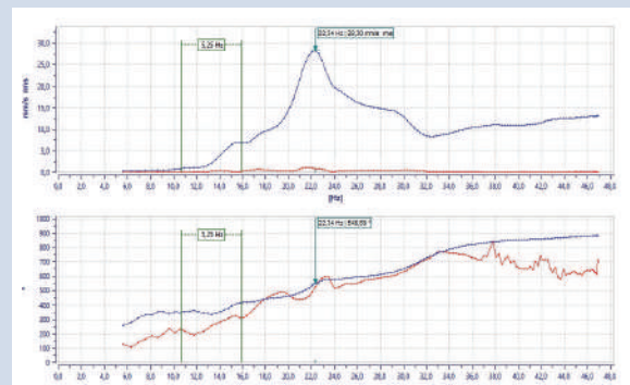
График Боде пуска агрегата
