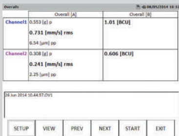
Двухканальные измерения общего уровня вибрации (полос. Фильтр VCU)
