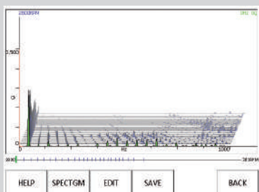
Водопадный график спектра
