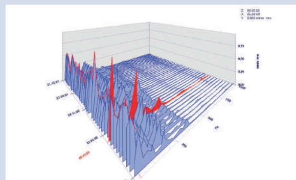
Водопадный график БПФ
