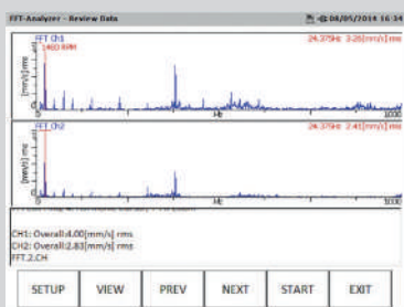
Двухканальный спектр
