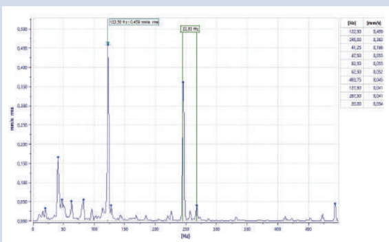
БПФ спектр
