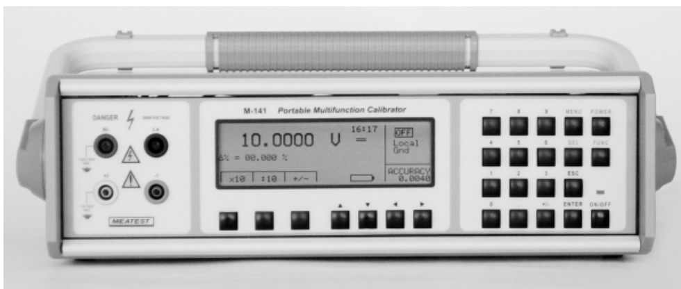
Рисунок 2 – Фотография передней панели CALIBRO-141
