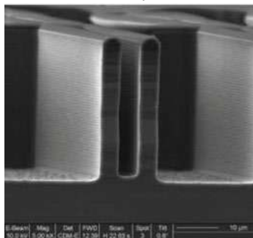
Кремний с вытравленными канавками
